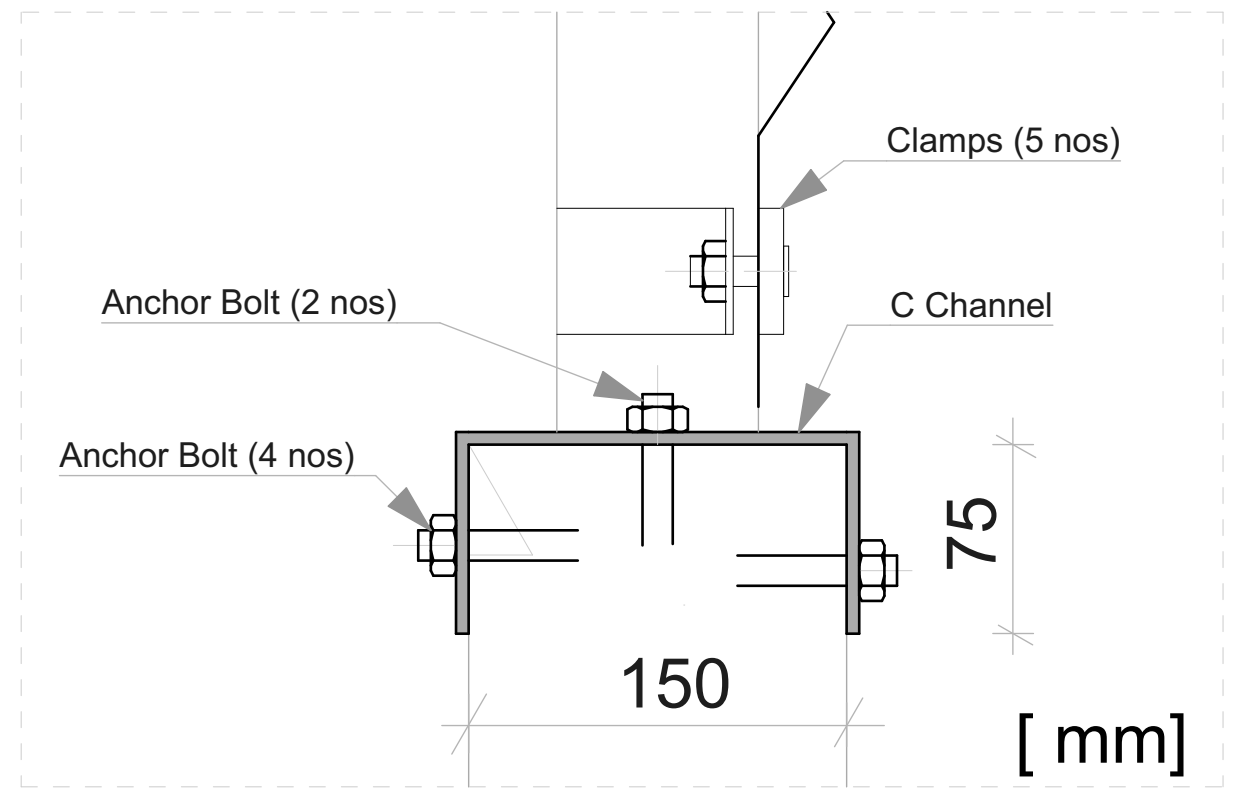
FIXING DETAIL D2
