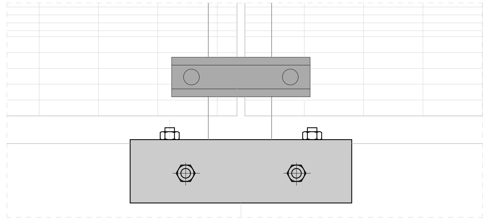
FIXING DETAIL D1
